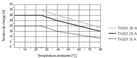
COURBES DE DÉPRÉCIATION TH201 15 ÷ 30A
