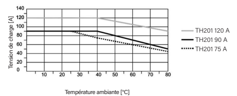
COURBES DE DÉPRÉCIATION TH201 75 ÷ 120A
