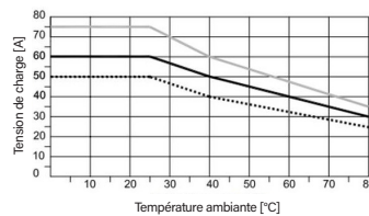
COURBES DE DÉPRÉCIATION TH201 40 ÷ 60A
